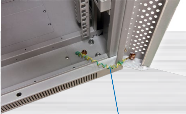
Erdungsverbindung Türe
